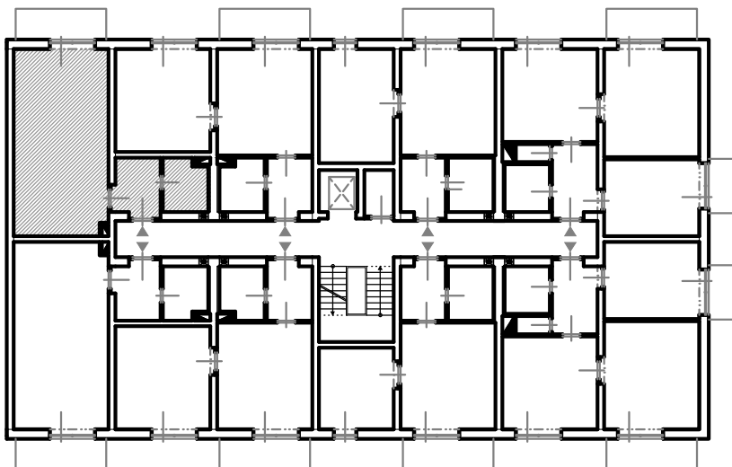
SCHÉMA PODLAŽÍ
