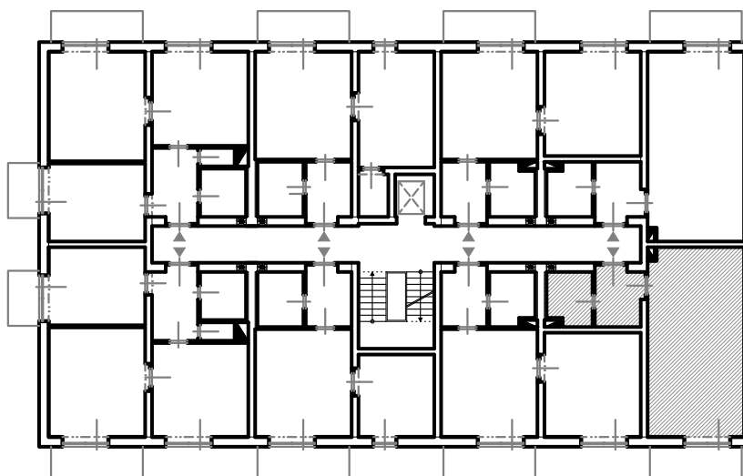
SCHÉMA PODLAŽÍ
